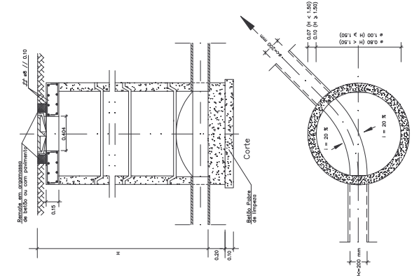
CAIXA DE RAMAL SIMPLES
